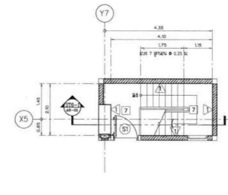
แบบขยายบันได ST-6 ชั้น 10 SCALE 1 : 75
