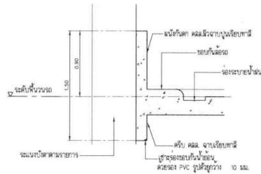
แบบขยาย E-02 SCALE 1 : 25
