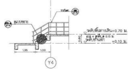
แบบขยายรูปตัดบันได ST3-1 SCALE 1 : 75
