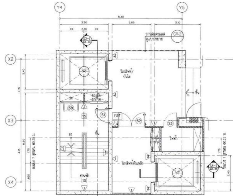
แบบขยายบันได ST-1 และลิฟต์ L3,L4 ชั้น 5-9 SCALE 1:75
