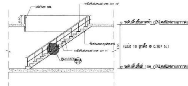
แบบขยายรูปตัดบันได ST7-1 SCALE 1 : 75
