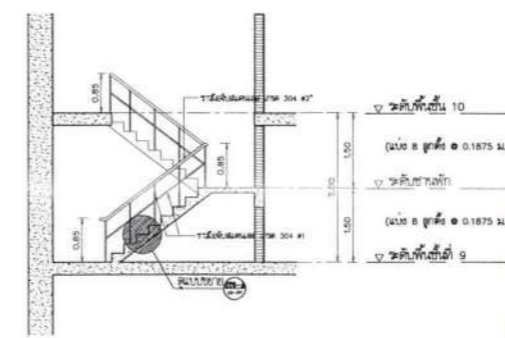
แบบขยายรูปตัดบันได ST6-1 SCALE 1 : 75
