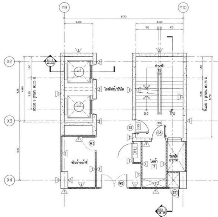
แบบขยายบันได ST-2 และลิฟต์ L1,L2 ชั้น 2-3 SCALE 1 : 75
