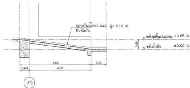
รูปตัดทางลาด R1-1 SCALE 1 : 75 R1-1 A6-08
