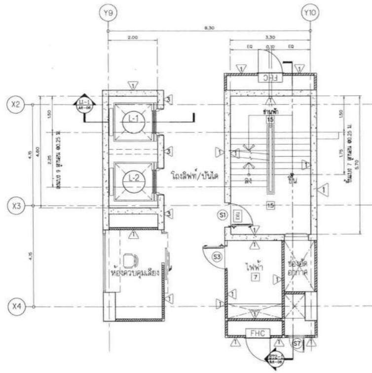
แบบขยายบันได ST-2 และลิฟต์ L1,L2 ชั้น 10- ชานพัก 2 SCALE 1 : 75
