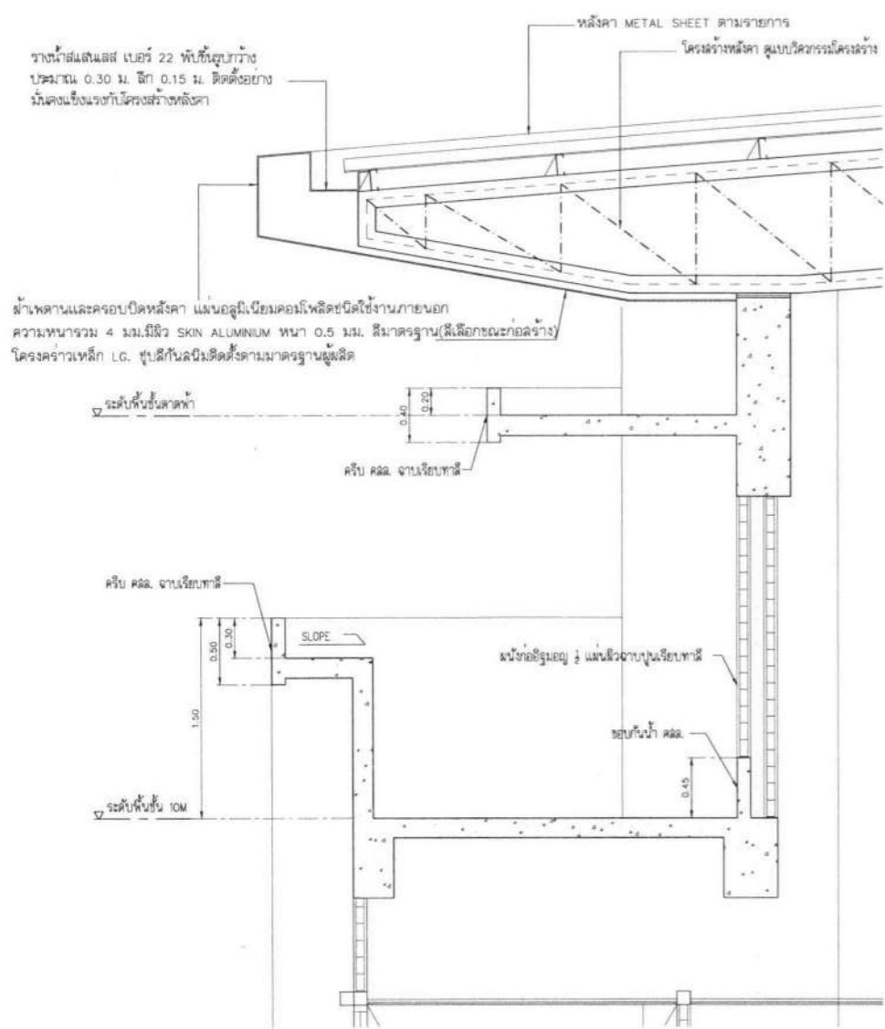
แบบขยาย C-04 SCALE 1 : 25
