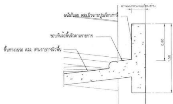
แบบขยาย A-09 SCALE 1 : 25
