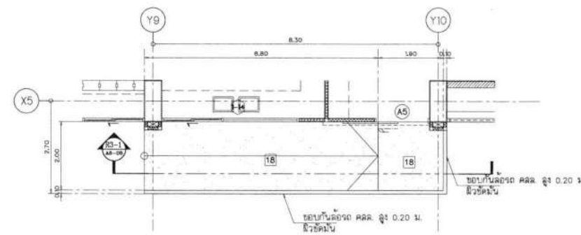
แบบขยายทางลาด R3 SCALE 1 : 75 R3 A6-08
