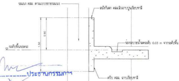
แบบขยาย B-03 SCALE 1 : 25
