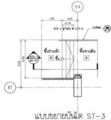
แบบขยายบันได ST-3 SCALE 1 : 75
