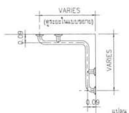
HR3 ราวพุงตัว สำหรับชักโครก (แบบพับแนวตั้ง) SCALE 1:20
