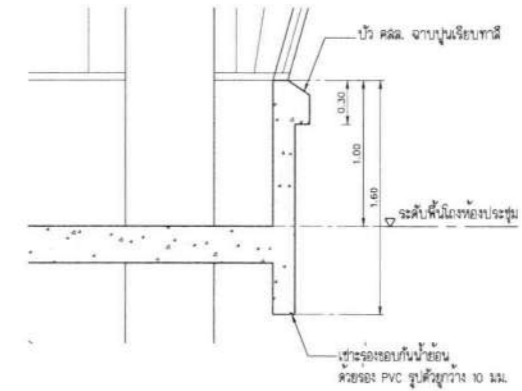
แบบขยาย A-08 SCALE 1 : 25
