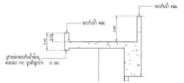
แบบขยาย E-03 SCALE 1 : 25
