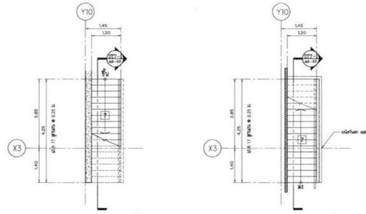
แบบขยายบันได ST-7 ชั้น 10M SCALE 1 : 75
