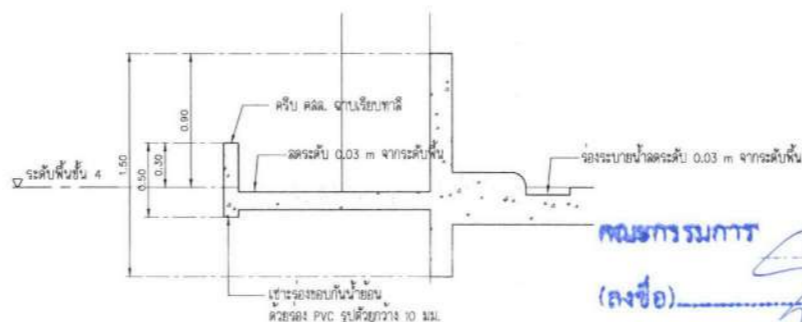
แบบขยาย B-02 SCALE 1 : 25
