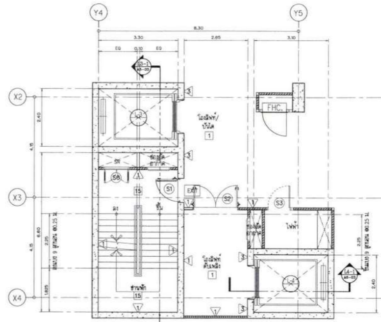
แบบขยายบันได ST-1 และลิฟต์ L3,L4 ชั้น 3-4 SCALE 1:75
