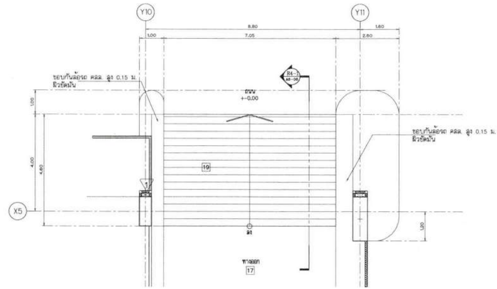
แบบขยายทางลาด R4 SCALE 1 : 75 R4 A6-08
