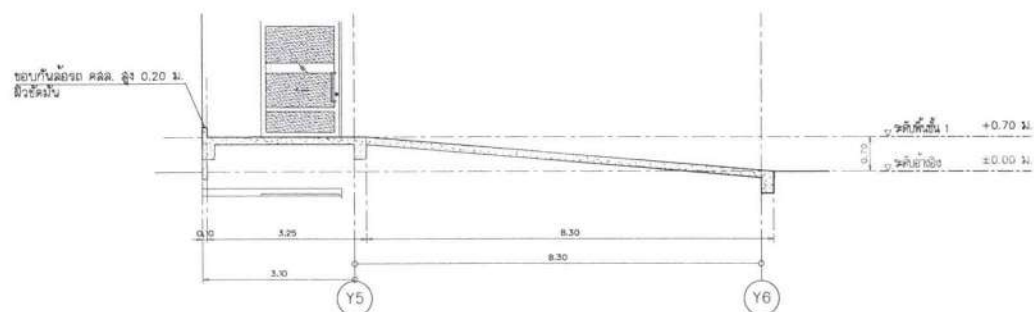
รูปตัดทางลาด R2-1 SCALE 1 : 75 R2-1 A6-08
