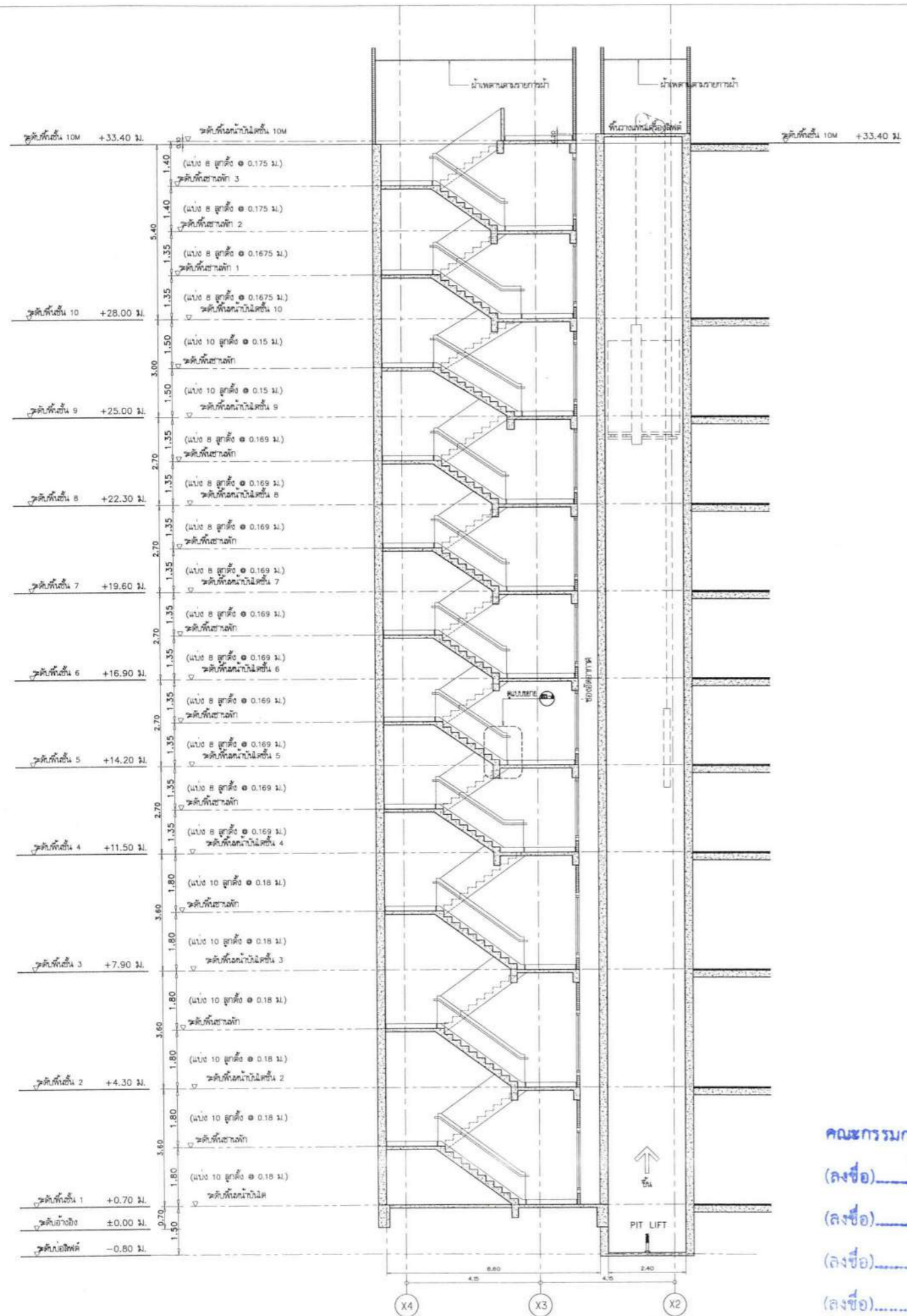
แบบขยายรูปตัดบันได STI-1 และแบบขยายรูปตัดลิฟต์ L3-1 SCALE 1 : 75
