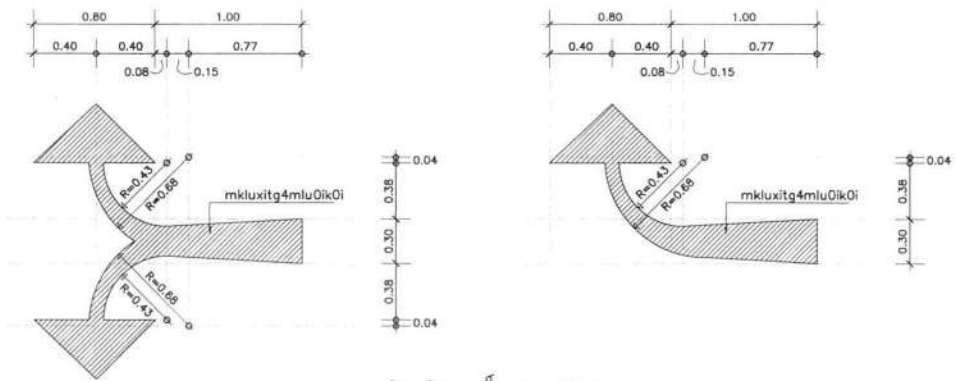
แบบขยายสัญลักษณ์แสดงทิศทางการจราจร มาตรฐาน 1 : 50
