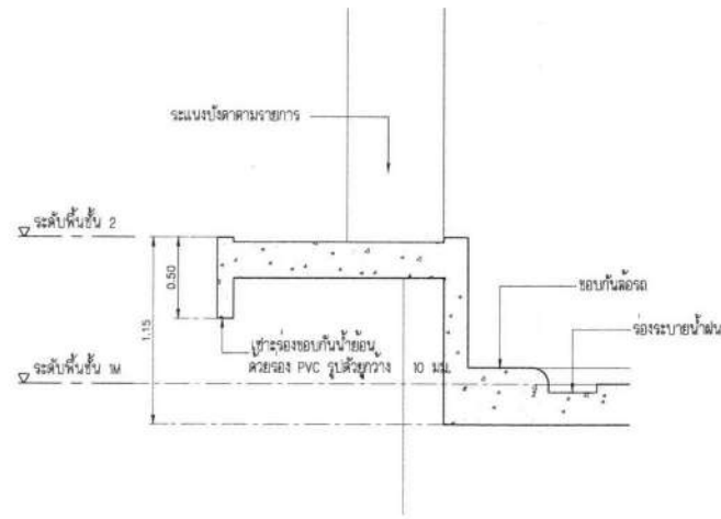
แบบขยาย E-01 SCALE 1 : 25
