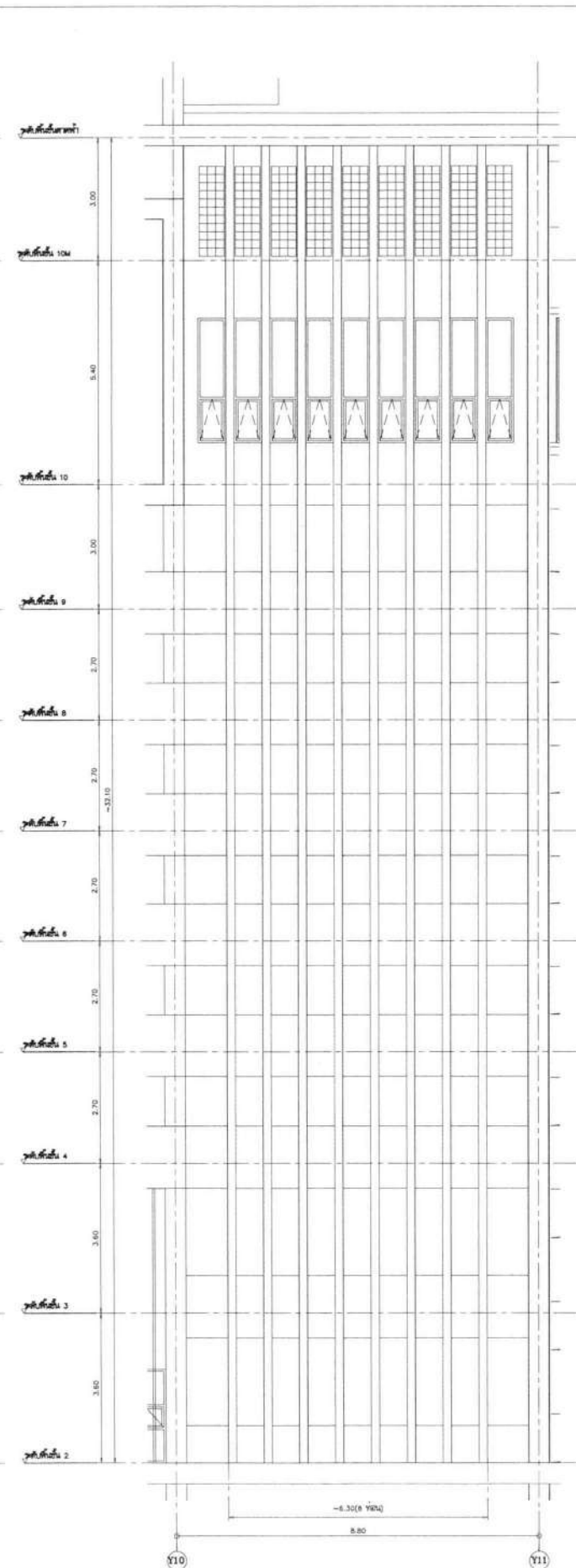
แบบขยาย G3-2 มาตราส่วน 1:75
