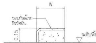
แบบขยายขอบกั้นล้อรถ มาตรฐาน 1 : หมายเหตุ W = ความกว้างรถรวมสองข้างแป้น
