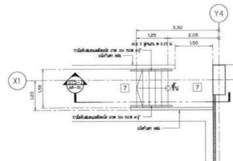
แบบขยายบันได ST-5 SCALE 1 : 75
