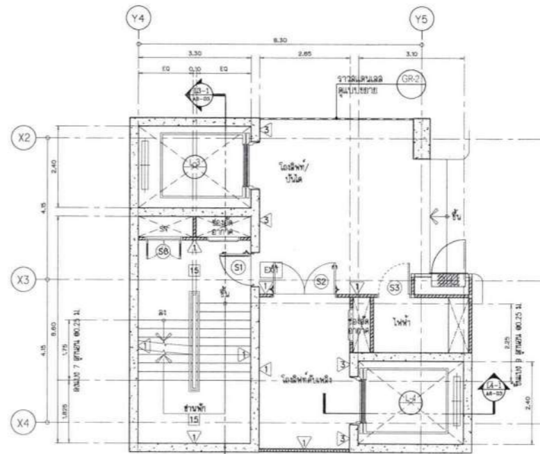
แบบขยายบันได ST-1 และลิฟต์ L3,L4 ชั้น 9-10 SCALE 1:75
