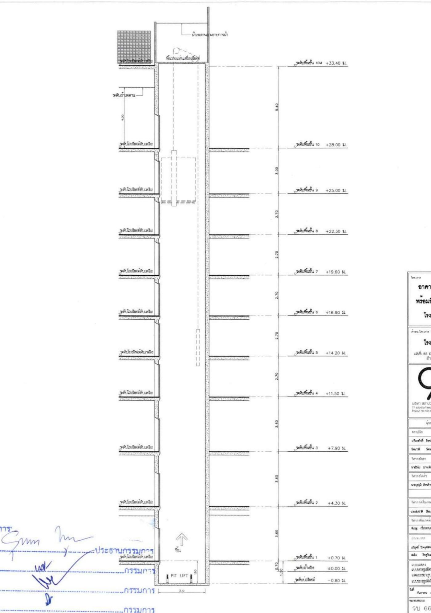
แบบขยายรูปตัดลิฟต์ L4-1 SCALE 1 : 75
