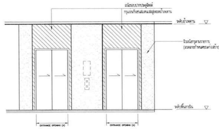
รูปตัดทางลิฟต์ L1,L2 SCALE 1 : 75
