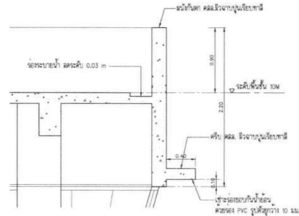
แบบขยาย A-07 SCALE 1 : 25
