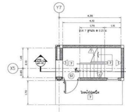
แบบขยายบันได ST-6 ชั้น 9 SCALE 1 : 75
