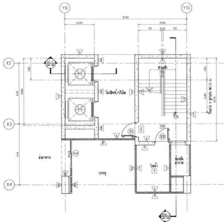
แบบขยายบันได ST-2 และลิฟต์ L1,L2 ชั้น 1-2 SCALE 1 : 75
