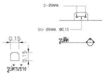
แบบขยาย ที่หยุดล้อรถ (WHEEL STOP) มาตรฐาน 1 : 50
