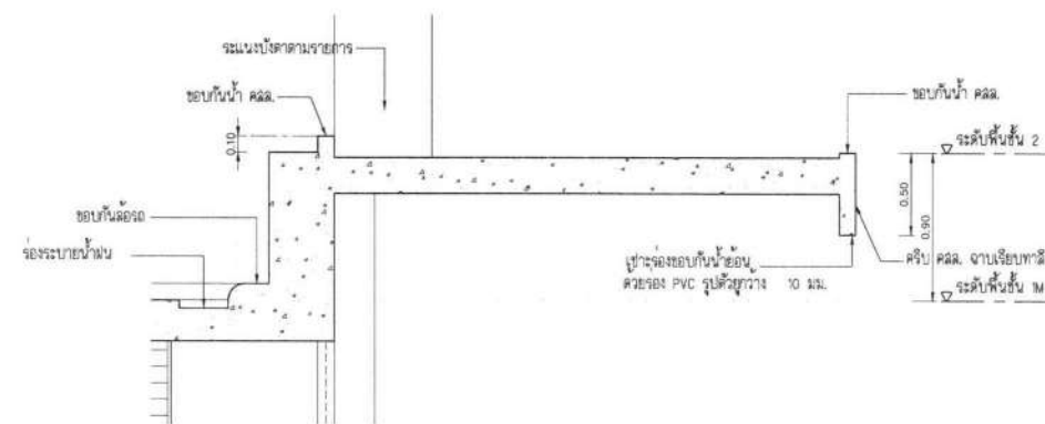
แบบขยาย E-06 SCALE 1 : 25
