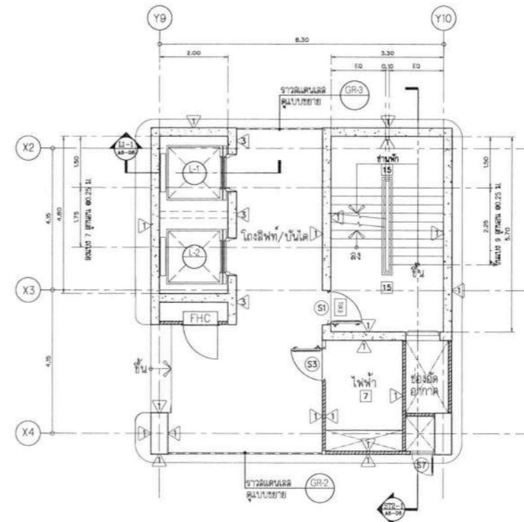
แบบขยายบันได ST-2 และลิฟต์ L1,L2 ชั้น 9-10 SCALE 1 : 75
