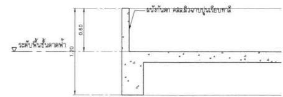
แบบขยาย A-04 SCALE 1 : 25
