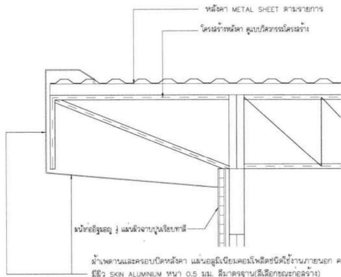
แบบขยาย A-05 SCALE 1 : 25
