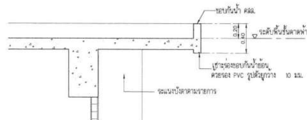
แบบขยาย E-05 SCALE 1 : 25
