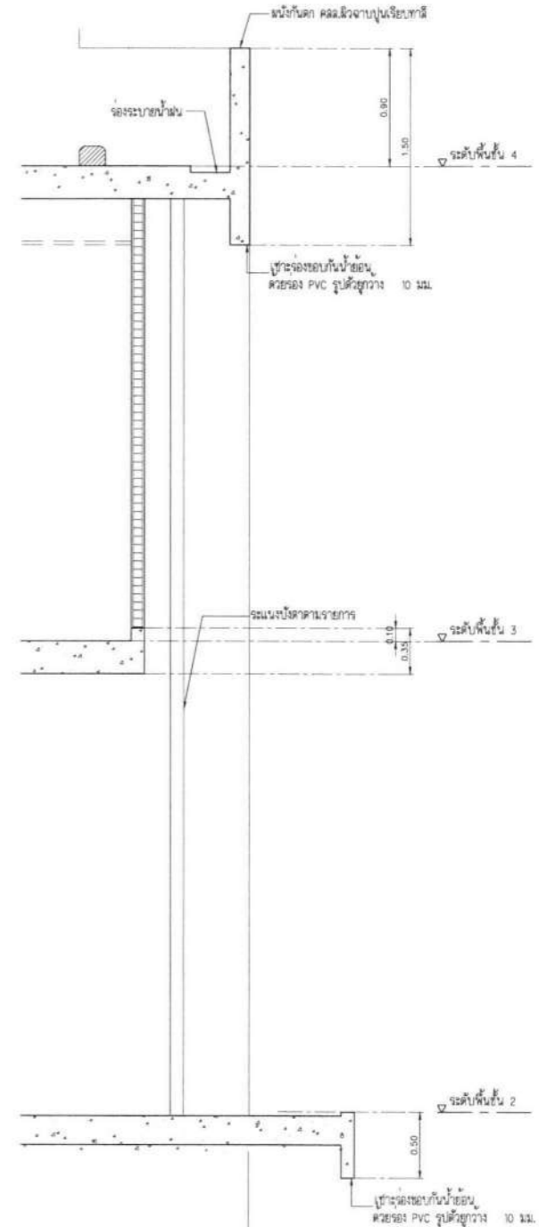
แบบขยาย C-06 SCALE 1 : 25
