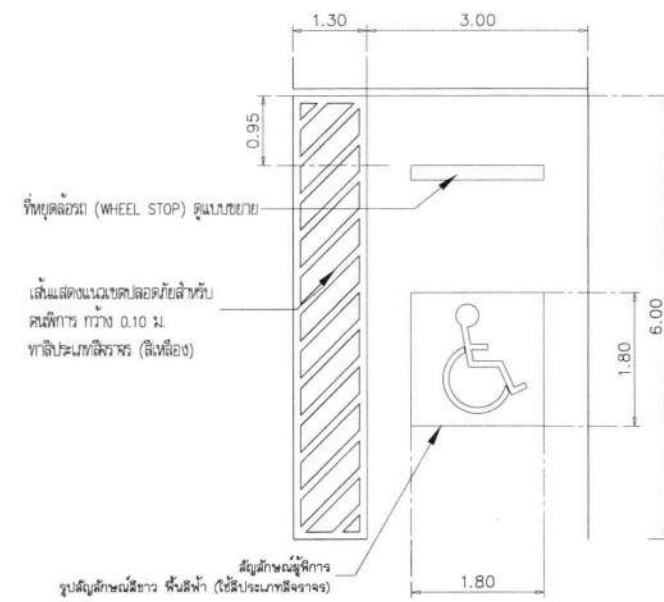
แบบขยาย การตีเส้นแบ่งแนวที่จอดรถผู้พิการ มาตรฐาน 1 : 50
