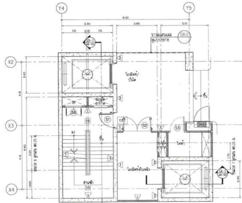
แบบขยายบันได ST-1 และลิฟต์ L3,L4 ชั้น 4-5 SCALE 1:75
