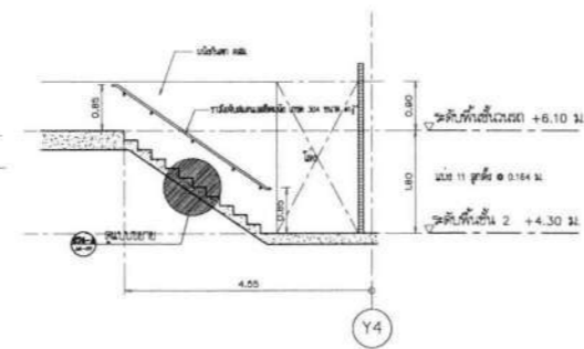
แบบขยายรูปตัดบันได ST4-1 SCALE 1 : 75
