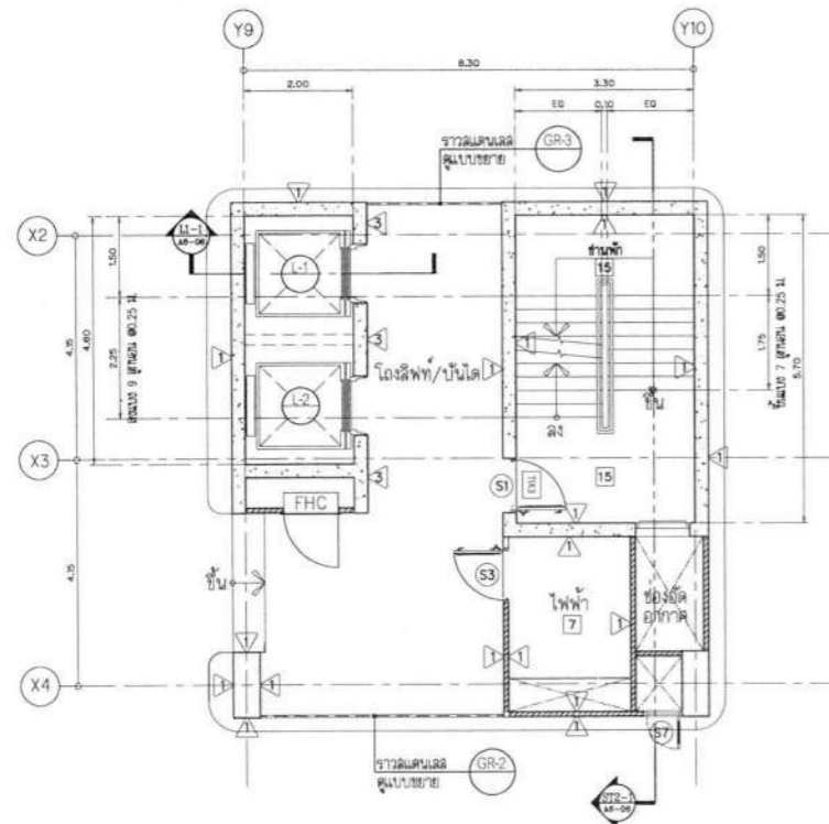
แบบขยายบันได ST-2 และลิฟต์ L1,L2 ชั้น 4-5 SCALE 1 : 75
