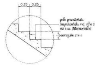
แบบขยายบันได ST4-A SCALE 1 : 12.5
