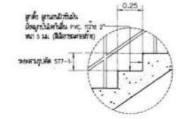
แบบขยายบันได ST7-A SCALE 1 : 12.5
