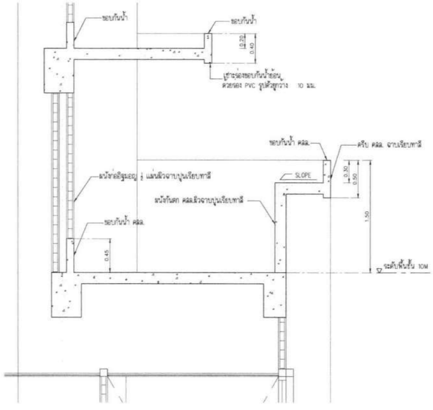
แบบขยาย C-05 SCALE 1 : 25
