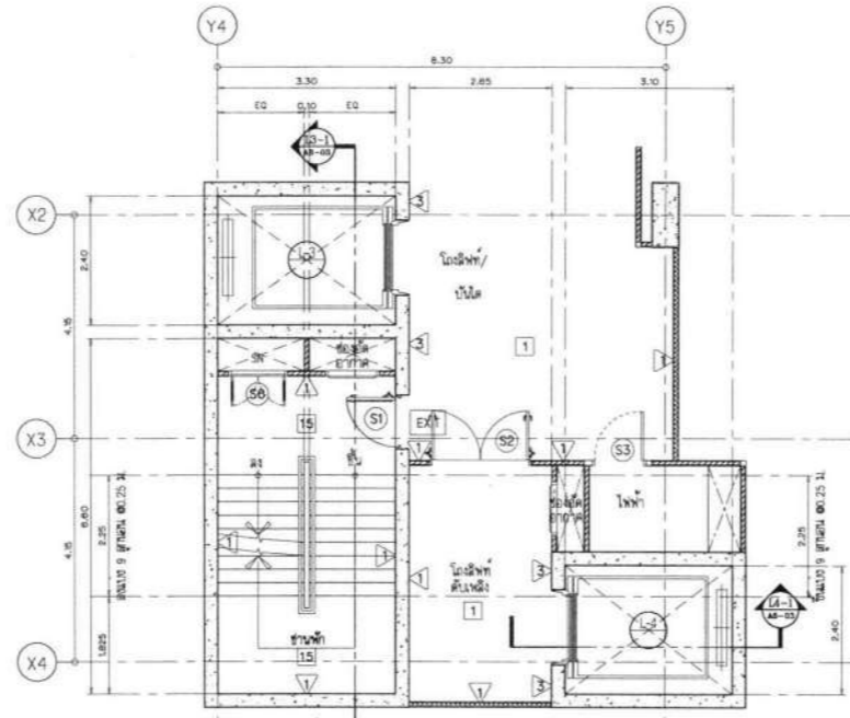
แบบขยายบันได ST-1 และลิฟต์ L3,L4 ชั้น 2-3 SCALE 1:75
