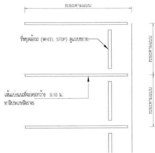
แบบขยาย การตีเส้นแบ่งแนวที่จอดรถ มาตรฐาน 1 : 50
