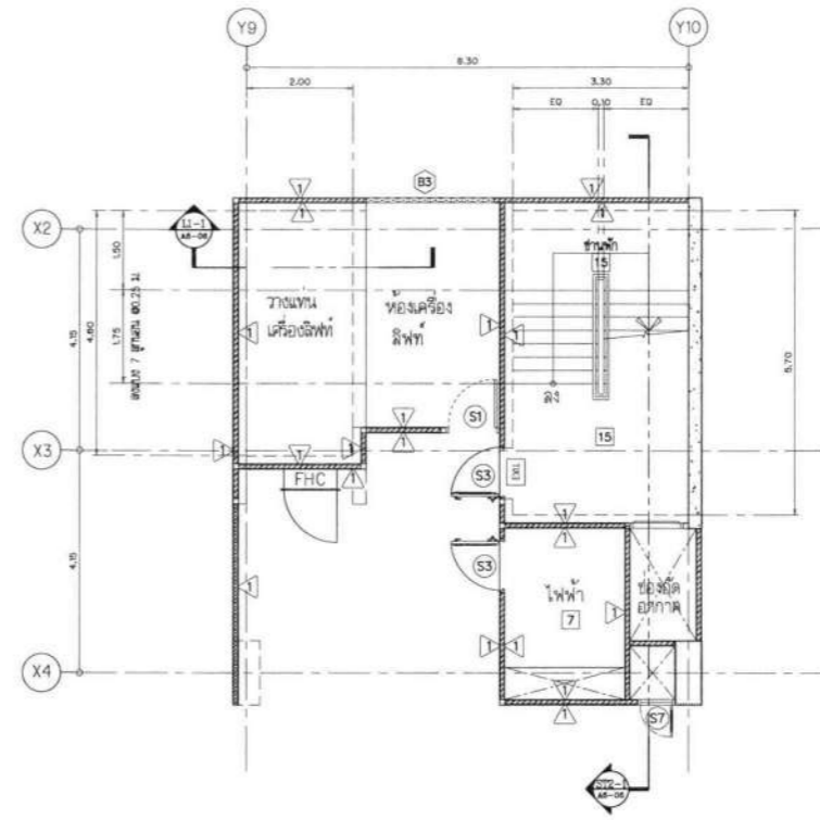
แบบขยายบันได ST-2 ชั้น 10M SCALE 1 : 75
