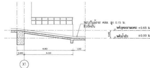
รูปตัดทางลาด R4-1 SCALE 1 : 75 R4-1 A6-08
