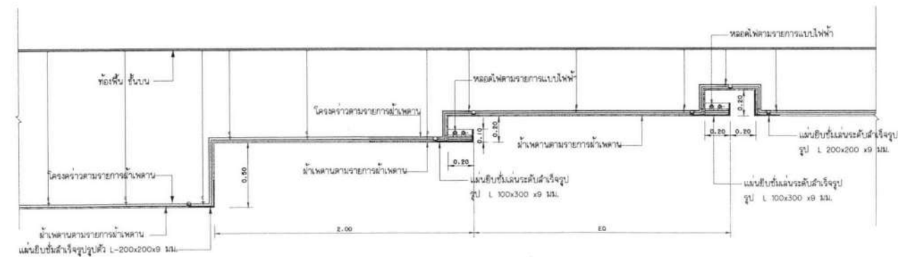
รูปตัดขยาย C1 มาตราส่วน 1 : 20
