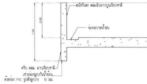
แบบขยาย D-02 SCALE 1 : 25
