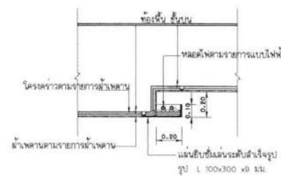
รูปตัดขยาย C2 มาตราส่วน 1 : 20
