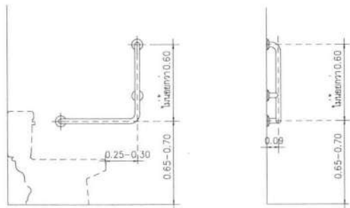
HR1 ราวพุงตัวรูปตัวแอล ชนิดติดผนังด้านขวา SCALE 1:20
