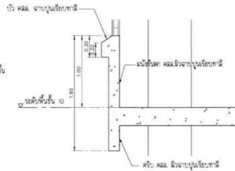
แบบขยาย A-02 SCALE 1 : 25
