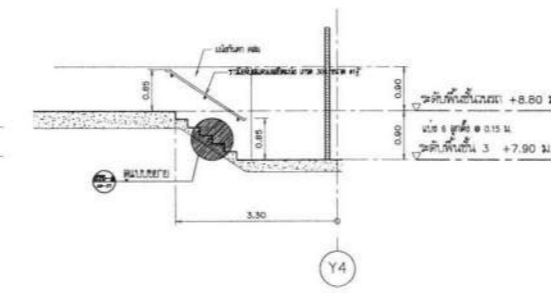
แบบขยายรูปตัดบันได ST5-1 SCALE 1 : 75
