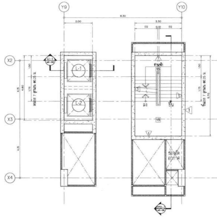
แบบขยายบันได ST-2 และลิฟต์ L1,L2 ชานพัก 2-ชั้น 10M SCALE 1 : 75
