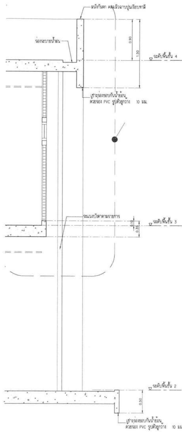
แบบขยาย D-05 SCALE 1 : 25
