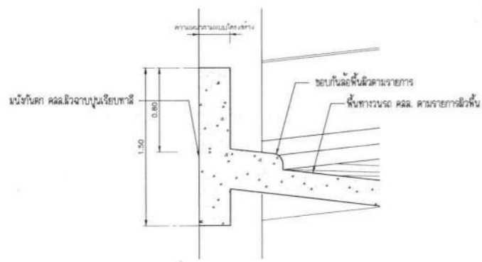
แบบขยาย A-01 SCALE 1 : 25
