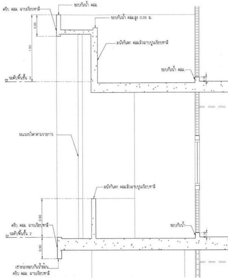
แบบขยาย D-01 SCALE 1 : 25
