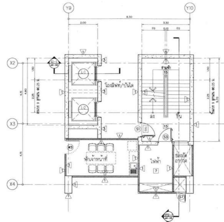
แบบขยายบันได ST-2 และลิฟต์ L1,L2 ชั้น 3-4 SCALE 1 : 75
