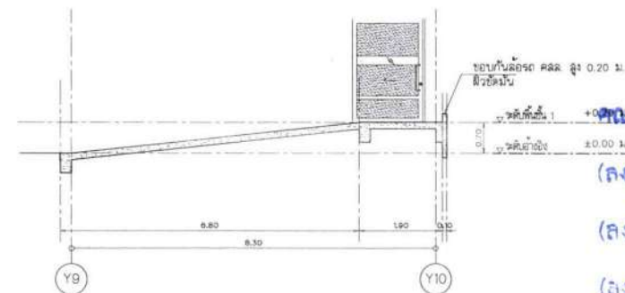
รูปตัดทางลาด R3-1 SCALE 1 : 75 R3-1 A6-08
