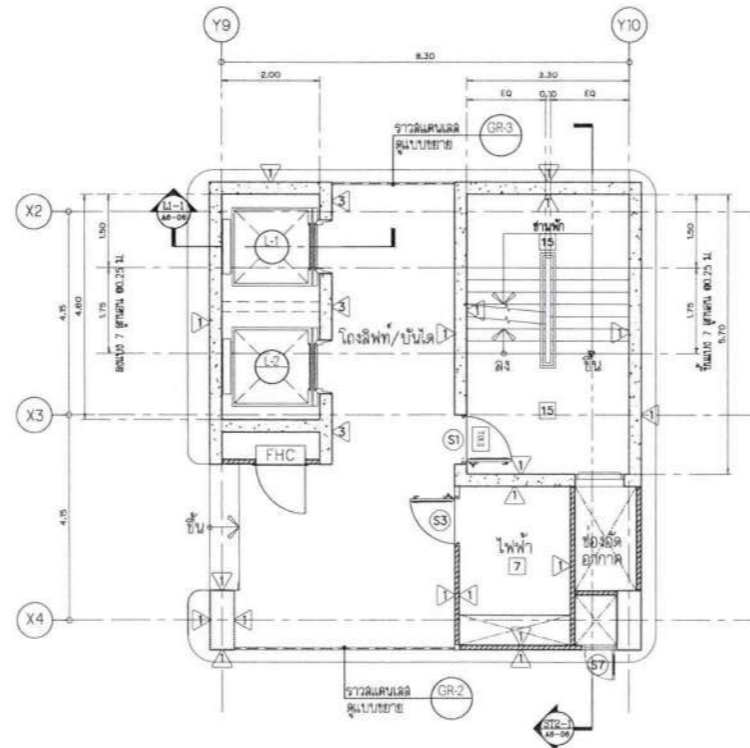
แบบขยายบันได ST-2 และลิฟต์ L1,L2 ชั้น 5-9 SCALE 1 : 75
