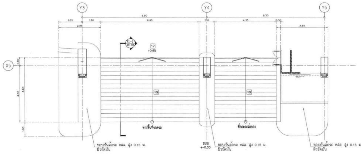
แบบขยายทางลาด R1 SCALE 1 : 75 R1 A6-08
