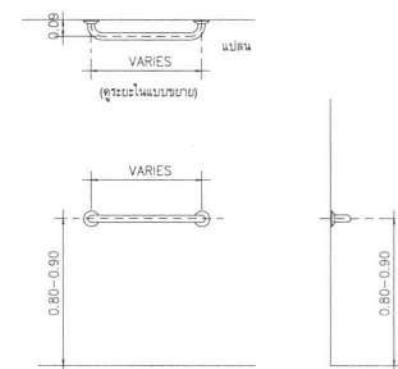
HR5 ราวพุงตัวแกว่งประแสง SCALE 1:20
