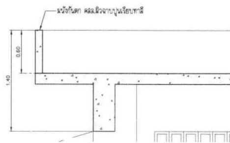
แบบขยาย E-04 SCALE 1 : 25
