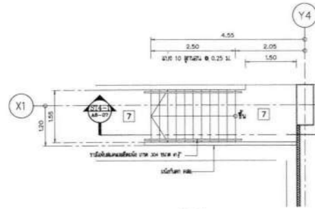
แบบขยายบันได ST-4 SCALE 1 : 75
