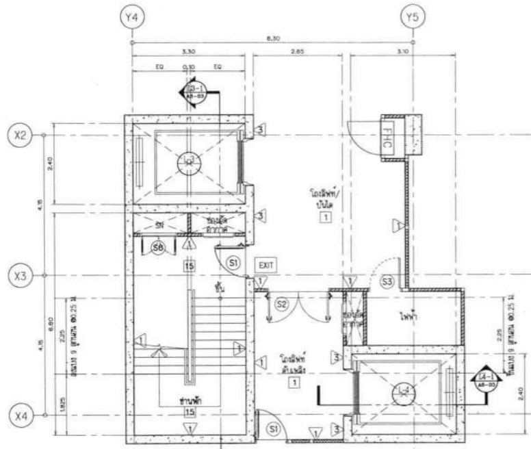
แบบขยายบันได ST-1 และลิฟต์ L3,L4 ชั้น 1 SCALE 1:75
